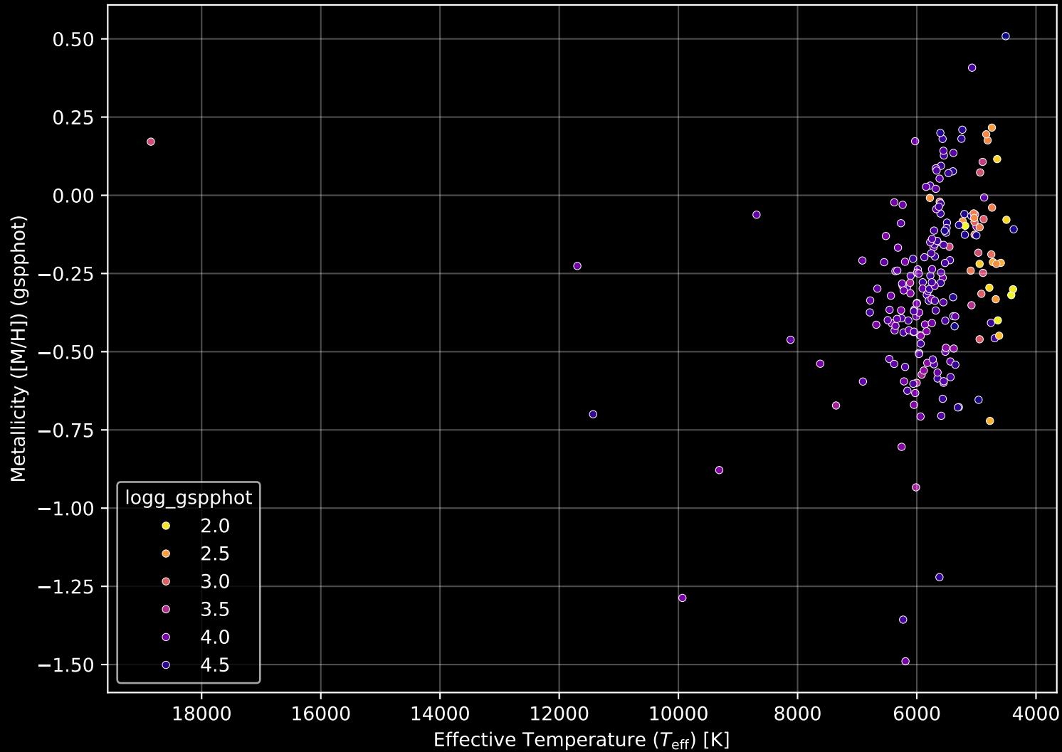
GALAH DR4 Field: [7152] Stellar Population Parameters (n= 209)
